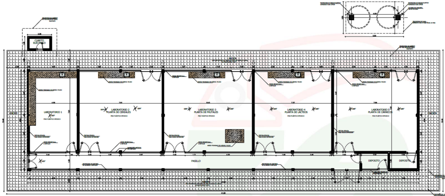
P LANTA ARQUITECTÓNICA PROPUESTA
